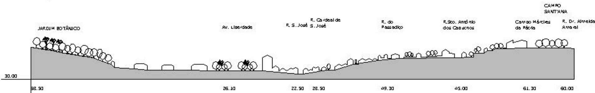
Carta de Morfologia do Terreno do Concelho de Lisboa
