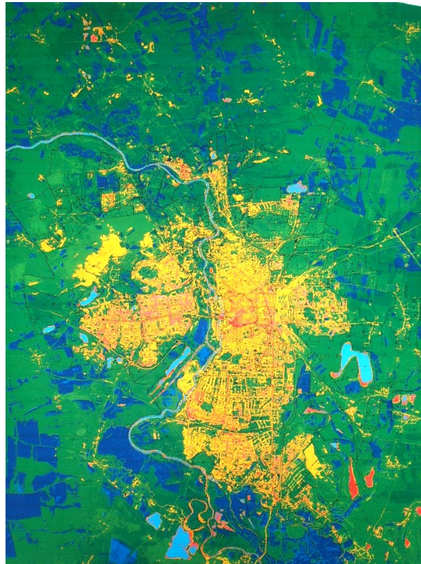
Carta de Topoclima Alemanha
