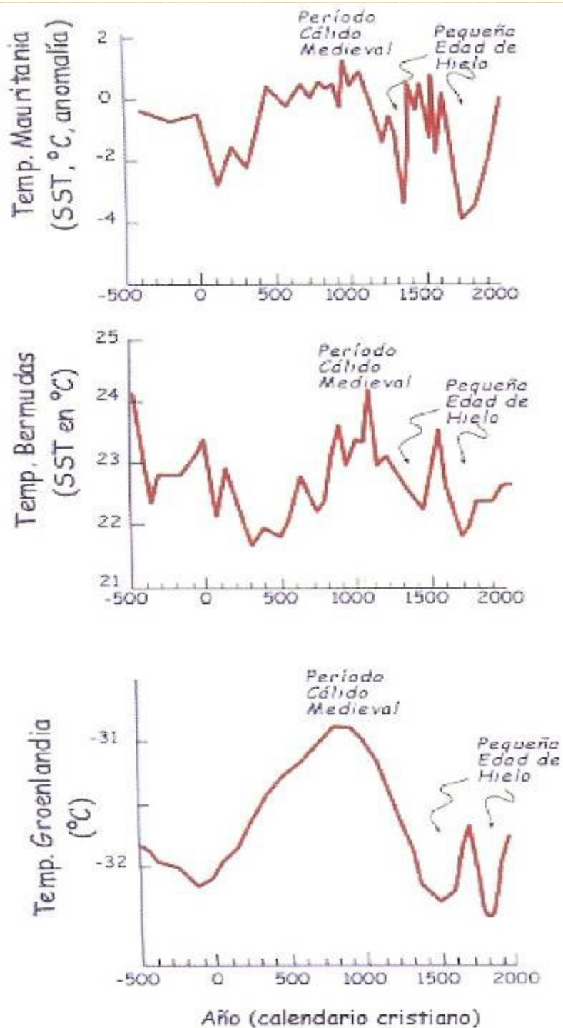
Figura 54. Evolución de las temperaturas superficiales del mar (sst) en los últimos 2.500 años en la costa de Mauritania (arriba) las Bermudas (en medio). Temperatura en Summit, Groenlandia (abajo). Se señalan el Período Cálido Medieval y la Pequeña Edad de Hielo, dividida en dos subperíodos.
