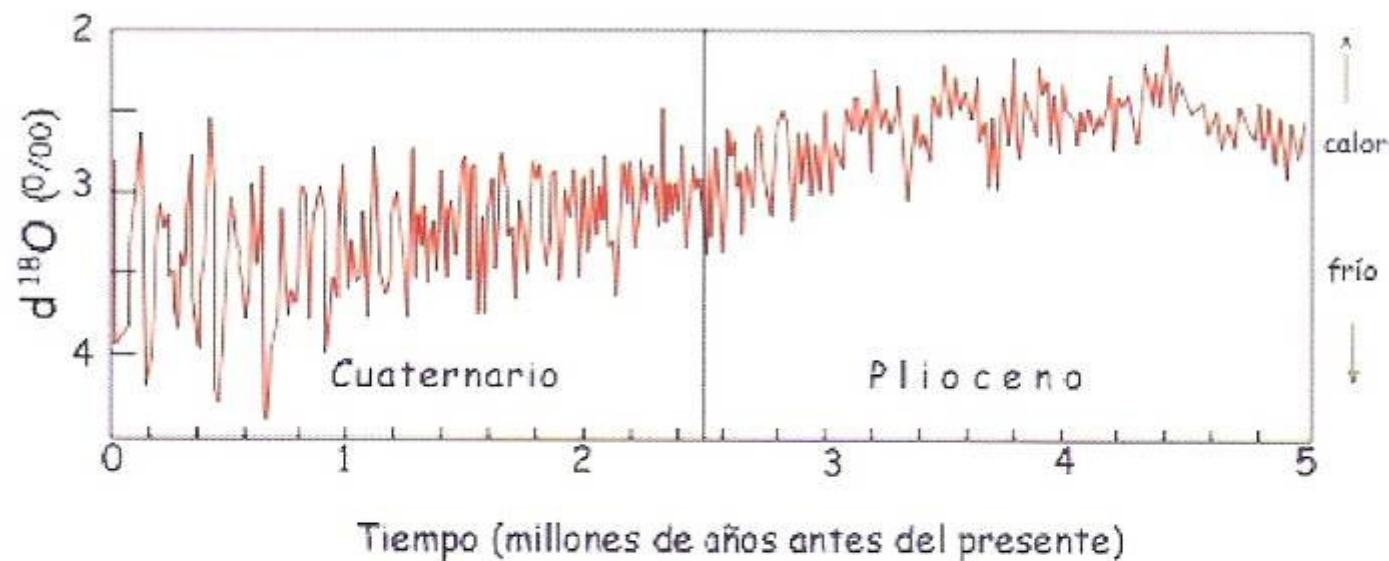
Figura 24. Plioceno y Cuaternario. Evolución de la concentración de oxígeno-18 en las conchas de los foraminíferos bénticos (de aguas profundas) durante los últimos 5 millones de años. La tendencia a un aumento de la concentración de oxígeno-18 (la escala está invertida) indica una tendencia general al frío y a una mayor acumulación de hielo en los continentes (ver dibujo explicativo). Obsérvese también el aumento de la oscilación térmica de los ciclos glaciales durante el Cuaternario, especialmente en el último millón de años. Los datos de \delta^{18}\text{O} son la media resultante en diversos sondeos del programa ODP (Ocean Drilling Project).
