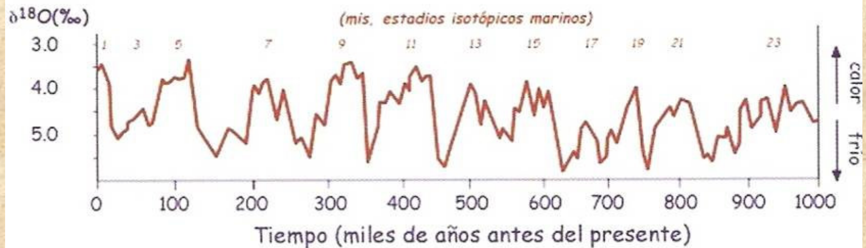
Figura 25. Glaciaciones cuaternarias. Ciclos glaciales en el último millón de años según el análisis isotópico del oxígeno de los foraminíferos (proyecto SPECMAP ). Se señalan también los estadios isotópicos marinos ( mis ). En los interglaciares cálidos disminuye la ratio isotópica del oxígeno-18 en el agua del mar y en las conchas de los foraminíferos (nótese que la escala vertical está invertida). En las glaciaciones aumenta.
