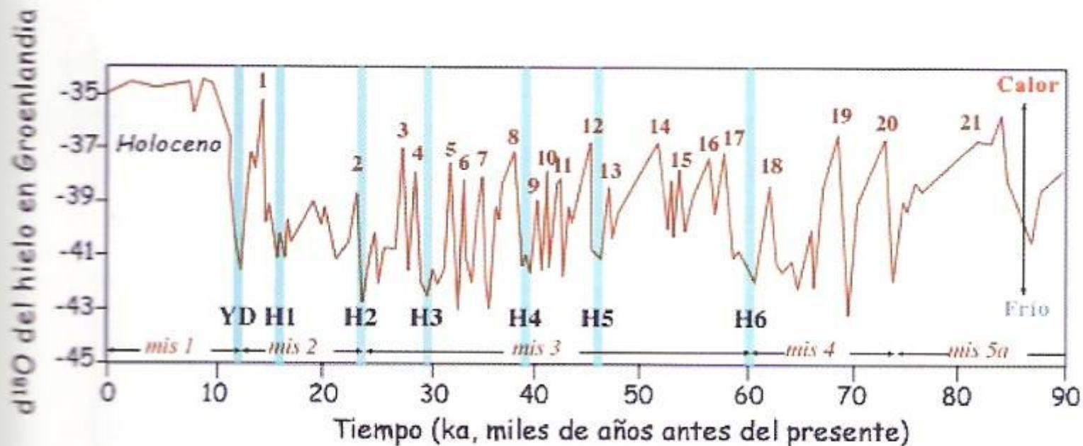
Figura 34. Inestabilidad climática durante la Última Glaciación según el sondeo GISP II de Groenlandia. Interestadales cálidos señalados con números y episodios Heinrich (suelta masiva de icebergs en el Atlántico Norte) con barras azules. Se señala también la compartimentación temporal en estadios isotópicos marinos (mis). YD es el último período frío: el Younger Dryas (ver mapas de circulación oceánica).
