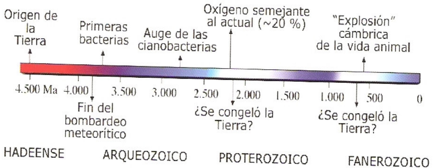
Figura 3. Algunos acontecimientos importantes de la historia de la Tierra.
