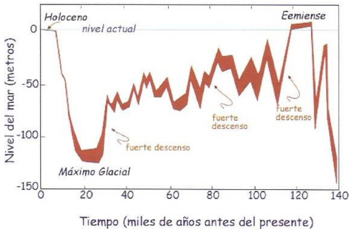
Figura 30. Nivel del mar durante los últimos 140 ka (miles de años) según las terrazas de coral de Huon (Nueva Guinea). Se señalan tres fases de descenso fuerte hacia el 115 ka, 85 ka y 30 ka aproximadamente. La anchura de la línea de variación indica la incertidumbre en el análisis.
