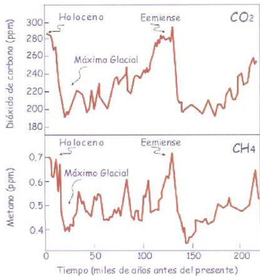
Figura 45. Concentración de dióxido de carbono (arriba) y de metano (abajo) durante el último ciclo glacial en partes por millón (ppm) del aire (fuente:sondeo GISP en Groenlandia).
