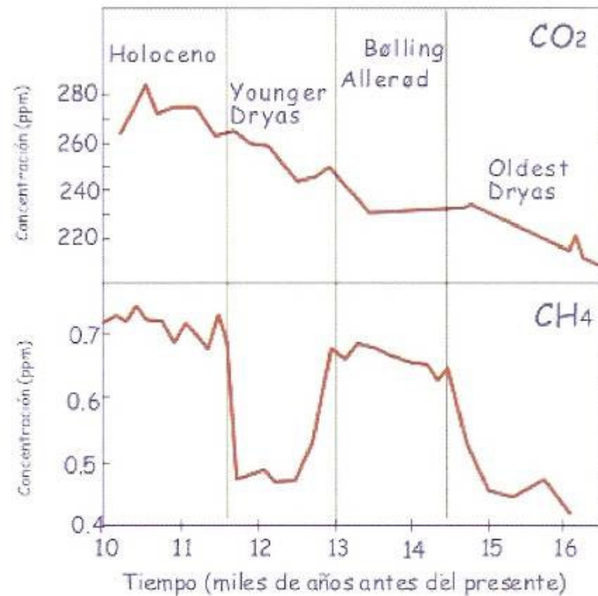
Figura 49. Evolución de las concentraciones de dióxido de carbono y de metano durante la última desglaciación. Durante el enfriamiento del Younger Dryas la concentración de dióxido de carbono (CO 2 ) no disminuyó, pero sí lo hizo la del metano (CH 4 ).
