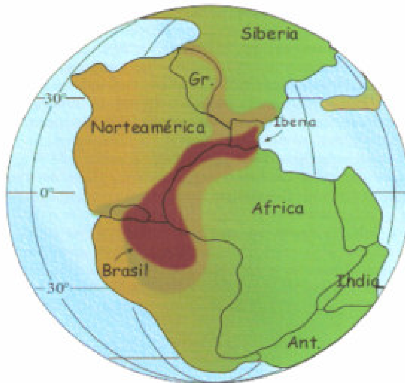
Figura 11. Final del Triásico y comienzo del Jurásico, hace 200 millones de años. Pangea comienza a dividirse entre Africa y América. Se denomina CAMP (Central Atlantic Magmatic Province) a la región de volcanes y de extrusión de coladas basálticas que llegaba desde Brasil hasta la Península Ibérica.
