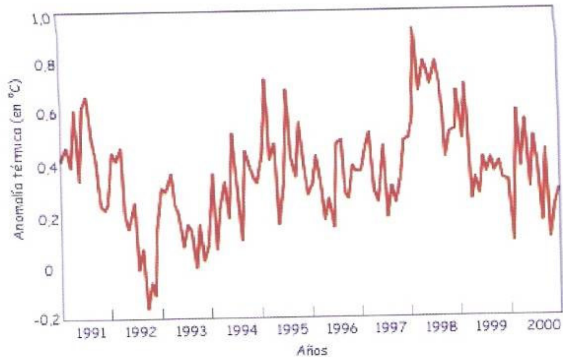
Figura 58. Detalle de la evolución térmica durante la década de los 90. Anomalías térmicas mensuales con respecto a la media del período 1951-1980 (fuente NASA). Se observa el bajón térmico tras la erupción del volcán Pinatubo en junio de 1991 y la subida del Niño en 1997-98.
