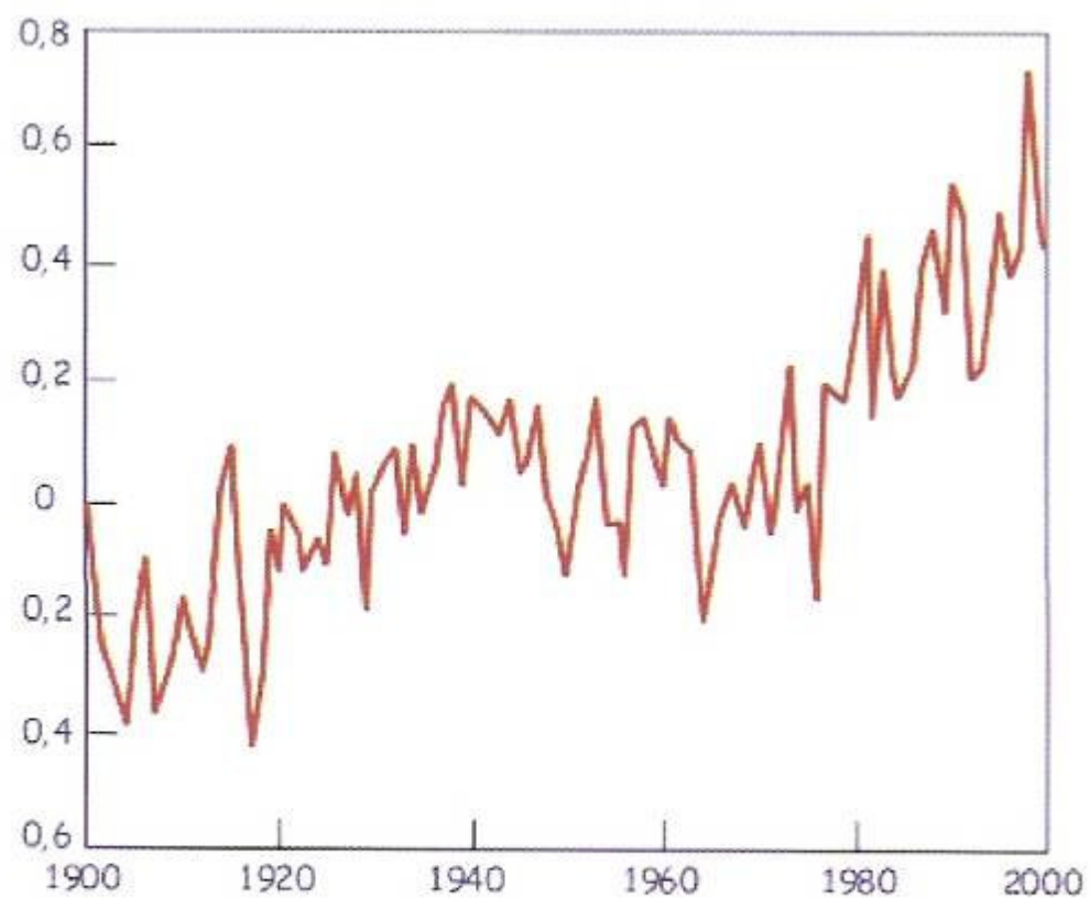
Figura 57. Evolución de la temperatura global media anual durante el siglo xx, a partir de termómetros de superficie, en °C. Se parte de un valor de referencia 0 en 1900 (fuente GISS).
