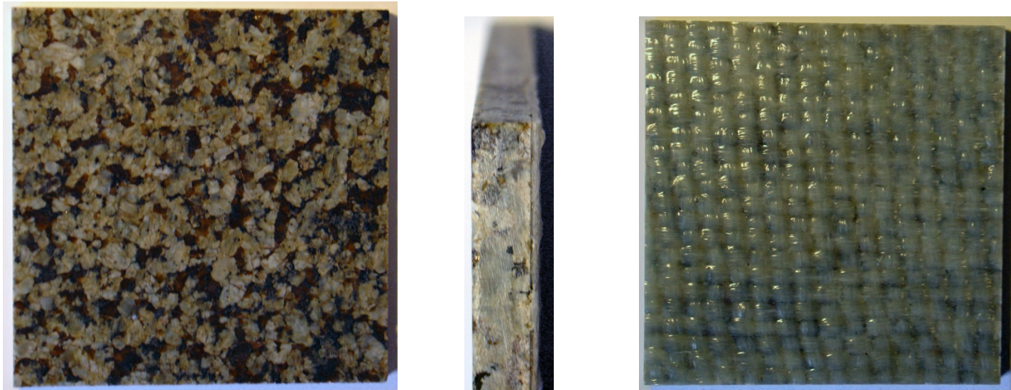
Fig.3 Placas de pedra natural reforçadas com malha de fibra de vidro e resina epóxi
